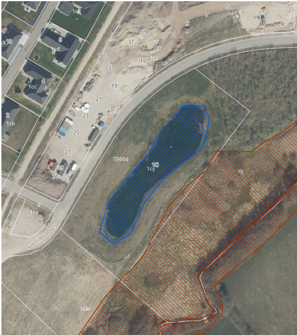
Oversigtskort over regnvandsbassin (markeret med blå) på Stenildvadvej 1C, 9600 Aars.
